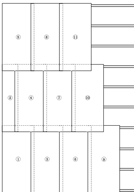
Versetzte Verlegung
