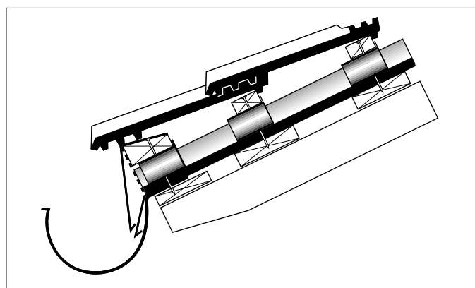
Hinterlüftung von Unterdach und Dacheindeckung
